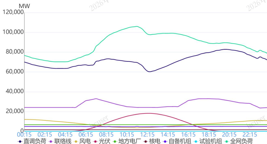
图1 6月29日负荷及电源出力预测情况
