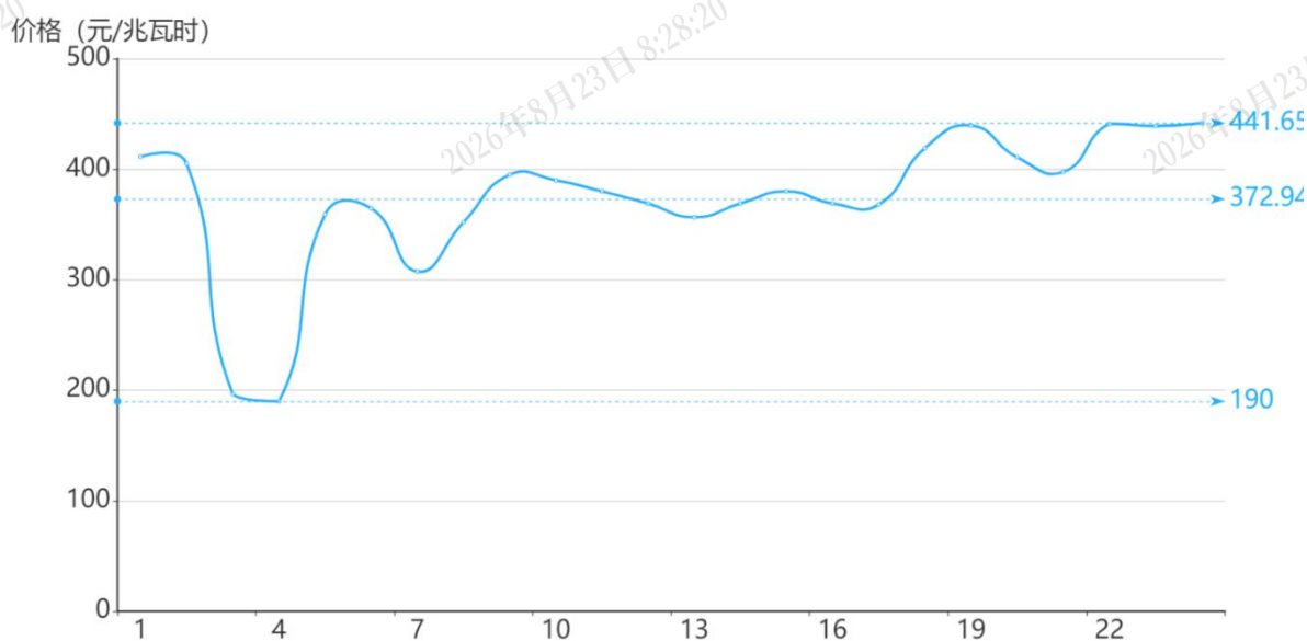
图 2 6 月 30 日日前市场用电侧价格
