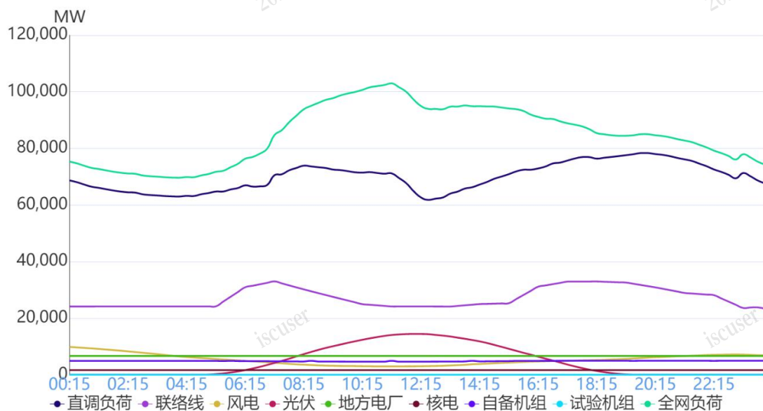
图1 6月30日负荷及电源出力预测情况
