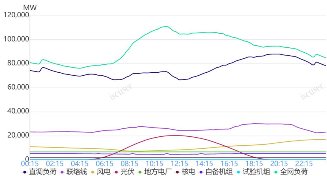
图 1 7 月 3 日负荷及电源出力预测情况
