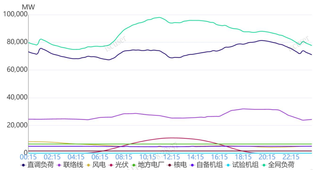
图 1 7月7日负荷及电源出力预测情况
