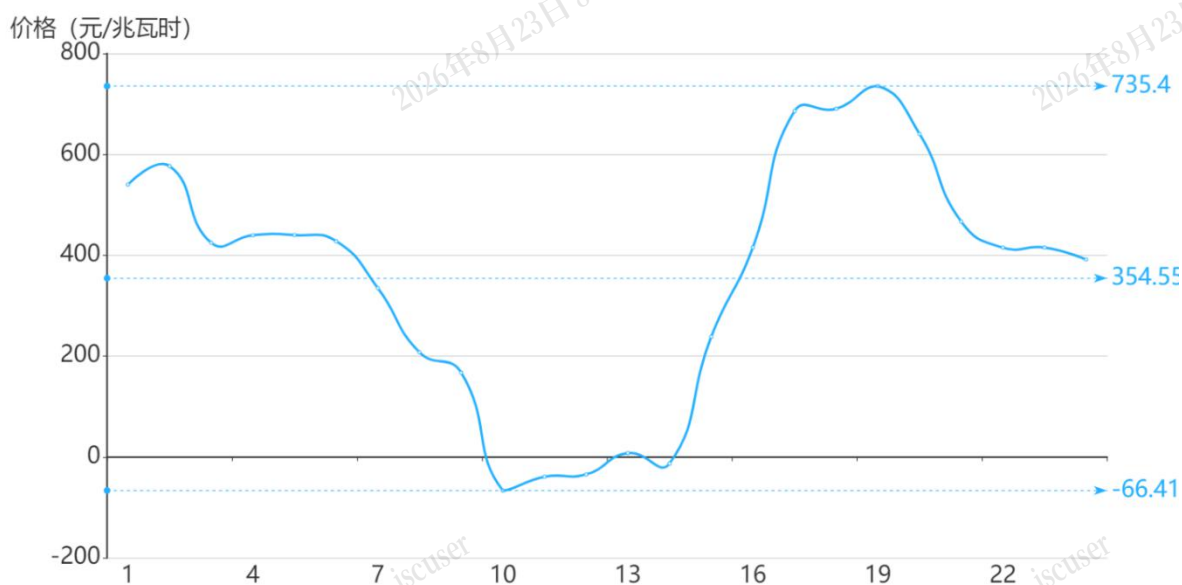
图 3 7 月 6 日实时市场用电侧价格
