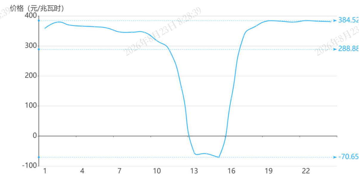
图 3 7 月 7 日实时市场用电侧价格
