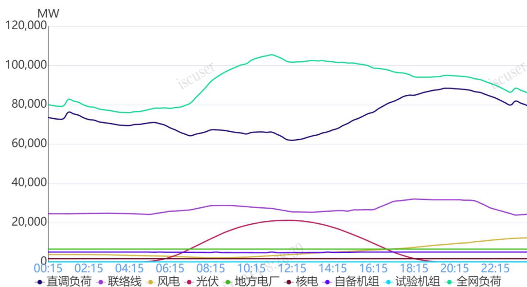
图 1 7月8日负荷及电源出力预测情况
