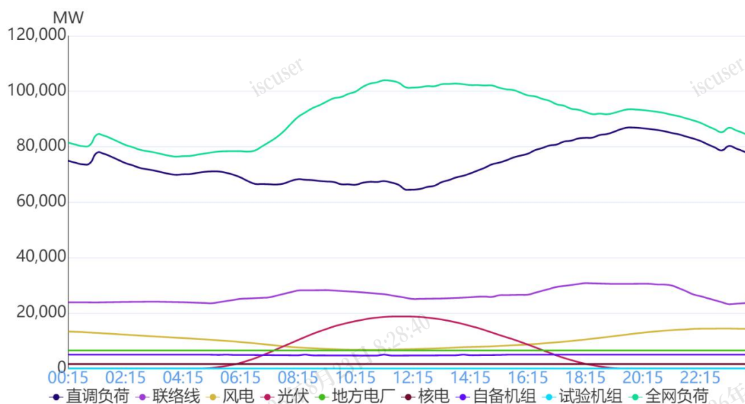
图 1 7月9日负荷及电源出力预测情况
