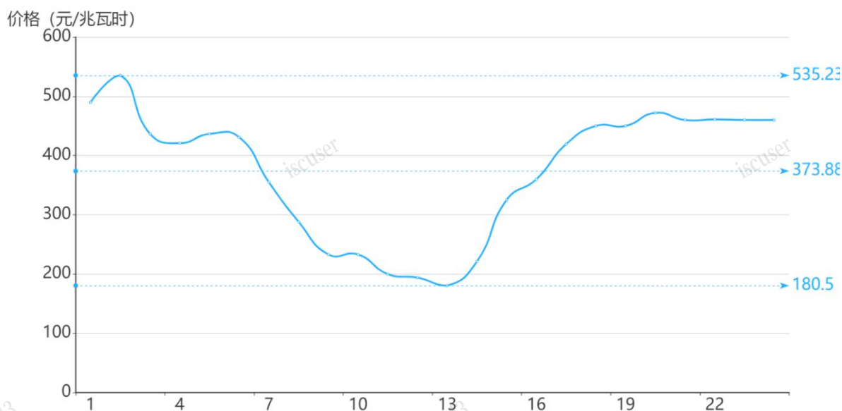
图2 7月10日日前市场用电侧价格
