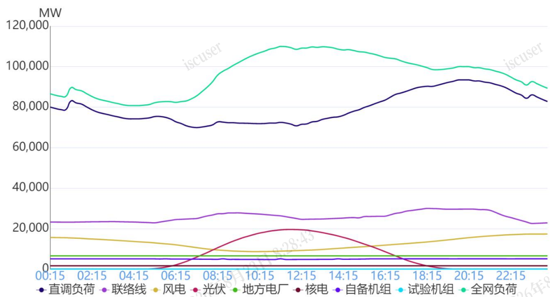
图 1 7月10日负荷及电源出力预测情况
