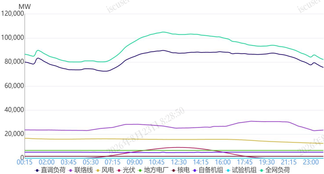
图1 7月13日负荷及电源出力预测情况
