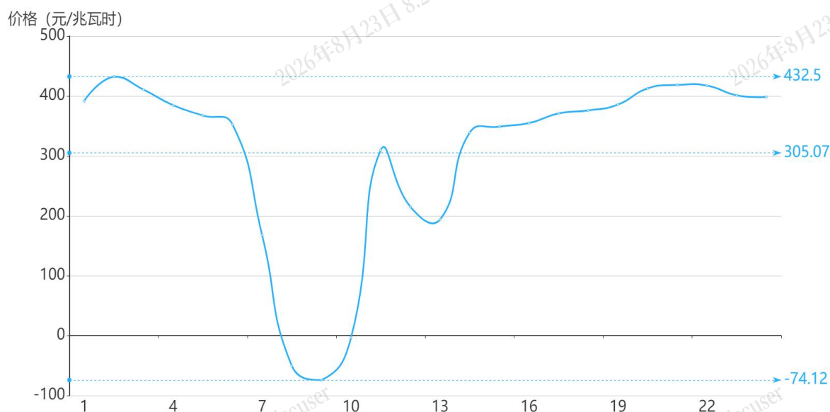
图 3 7 月 12 日实时市场用电侧价格
