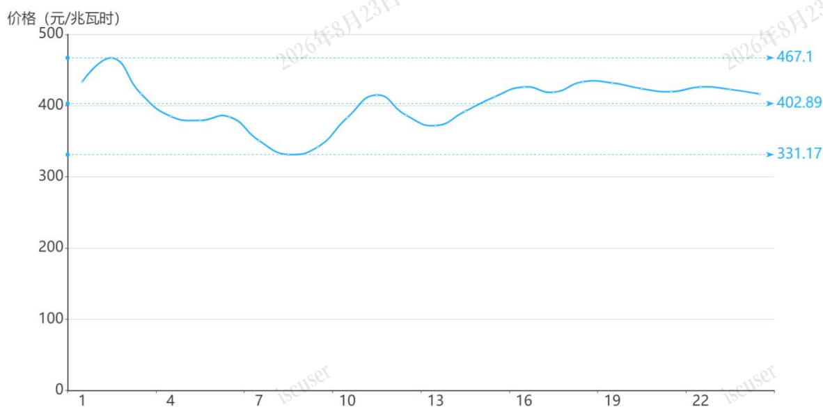
图3 7月27日实时市场用电侧价格
