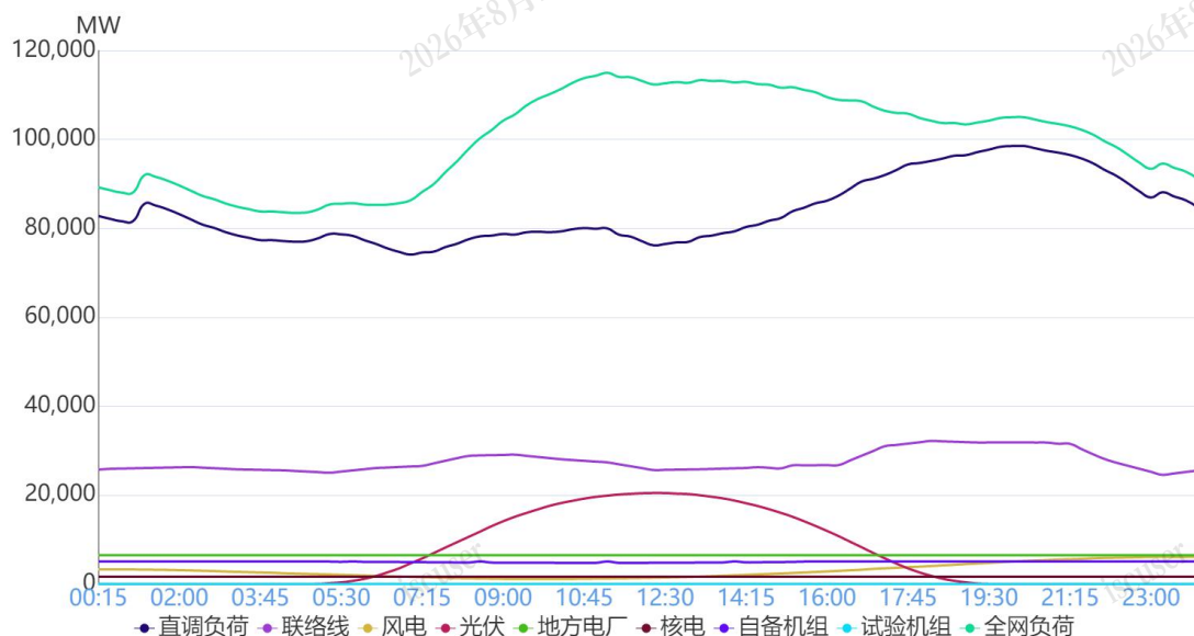
图 1 7月28日负荷及电源出力预测情况
