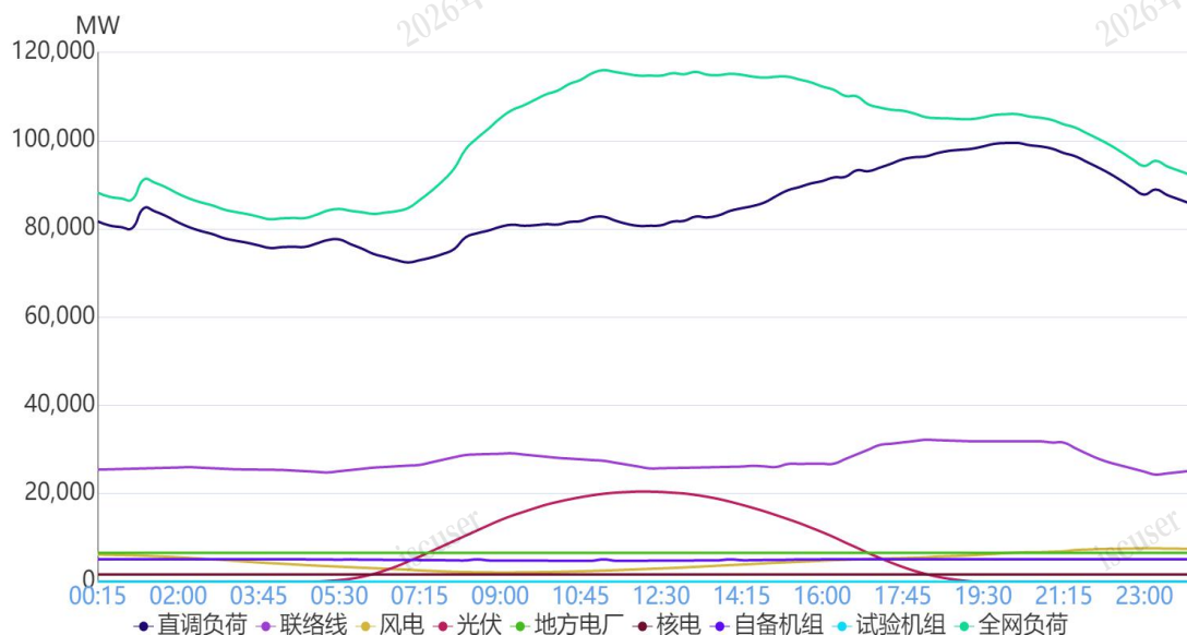
图 1 7月29日负荷及电源出力预测情况
