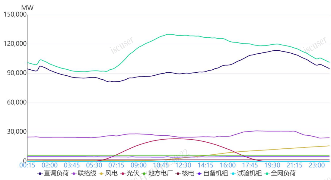
图 1 8月7日负荷及电源出力预测情况
