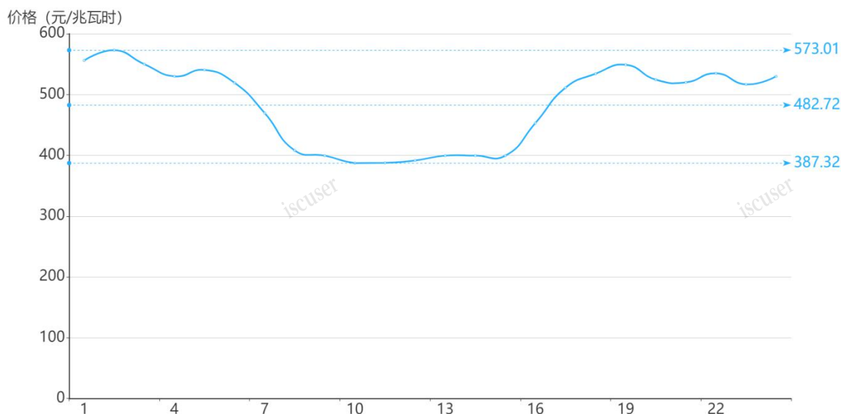
图2 8月7日日前市场用电侧价格
