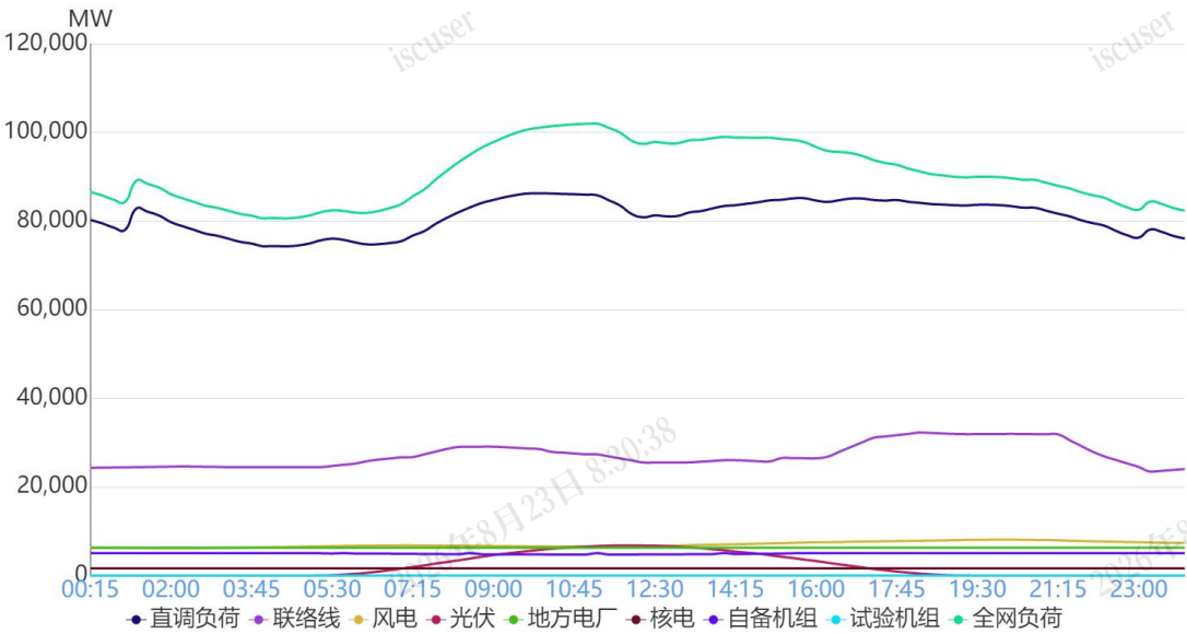
图 1 8月12日负荷及电源出力预测情况
