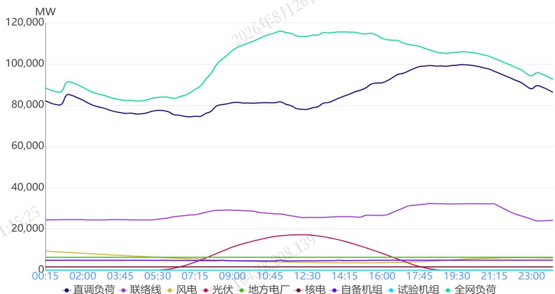
图 1 8月24日负荷及电源出力预测情况
