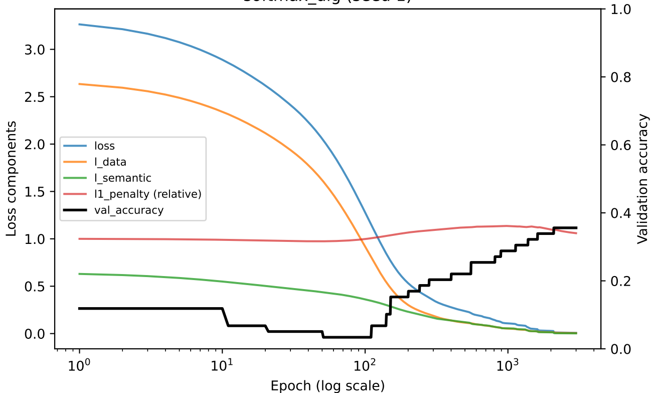
softmax_dlg (seed 1)
