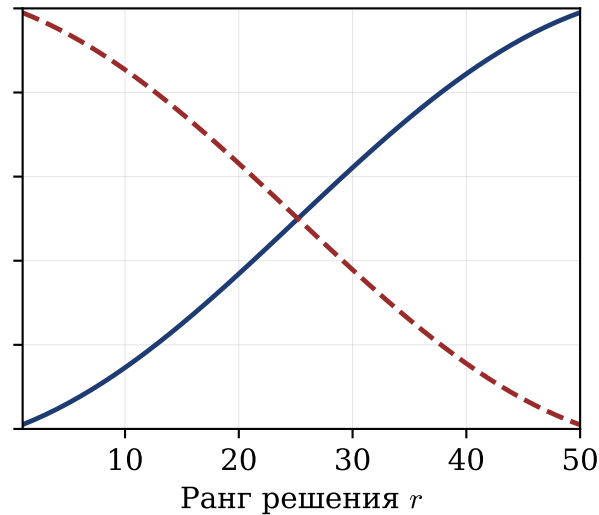
Смешанная модель, \alpha = 0,5
