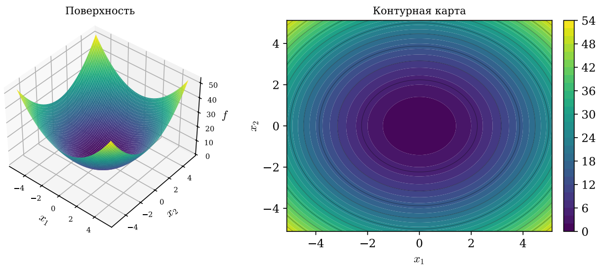
Рисунок 1 – Функция сферы: поверхность и контурная карта
