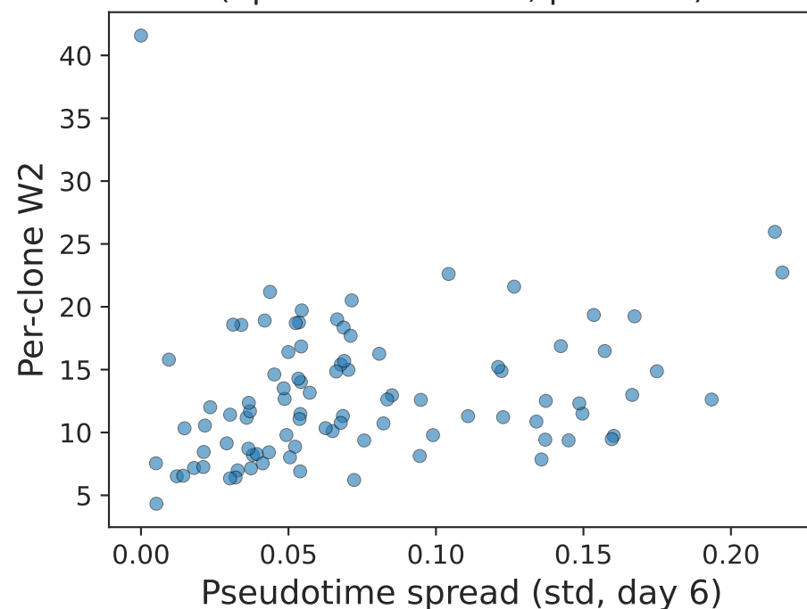
(d) W2 vs pseudotime spread (scDiffEq) (Spearman r=0.35 , p=0.001 )
