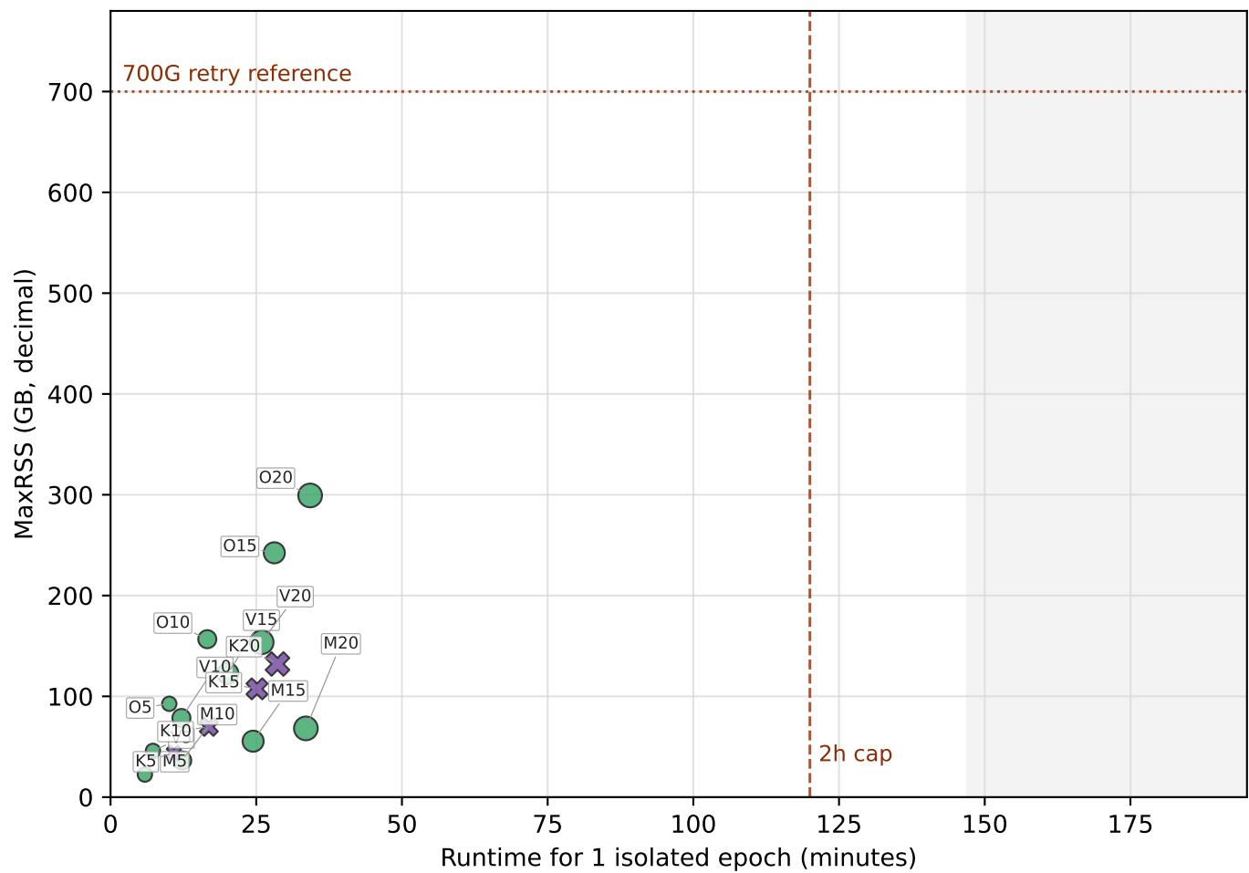
ProvBPF
