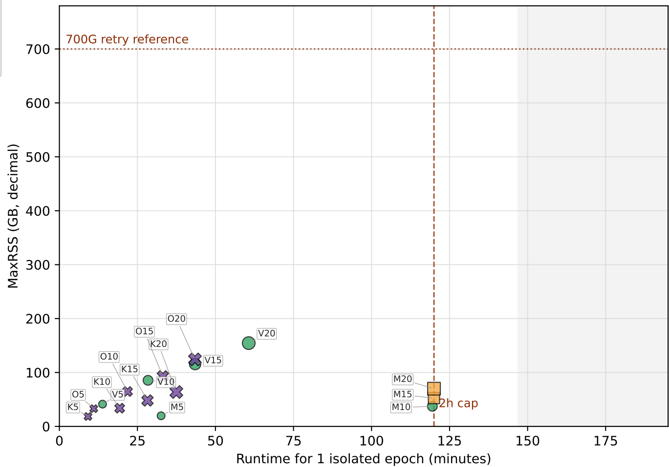
ConProv
