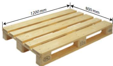
Euro-palette type I
