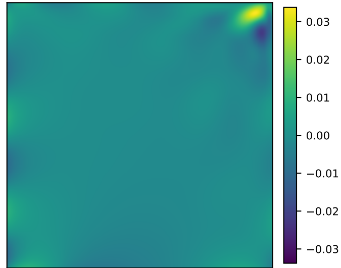
Error
