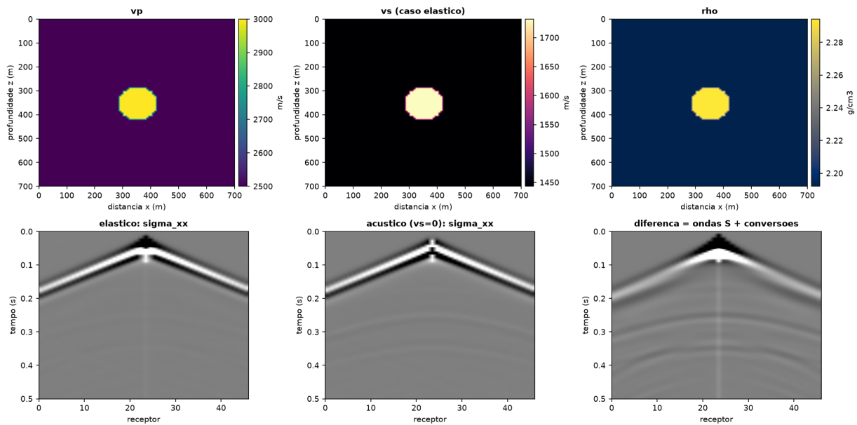
Figura 5.1: Prova do regime acústico. Pannel inferior direito: a diferença entre elástico e acústico são as ondas S e conversões P-S — com norma comparável à do próprio dado.
