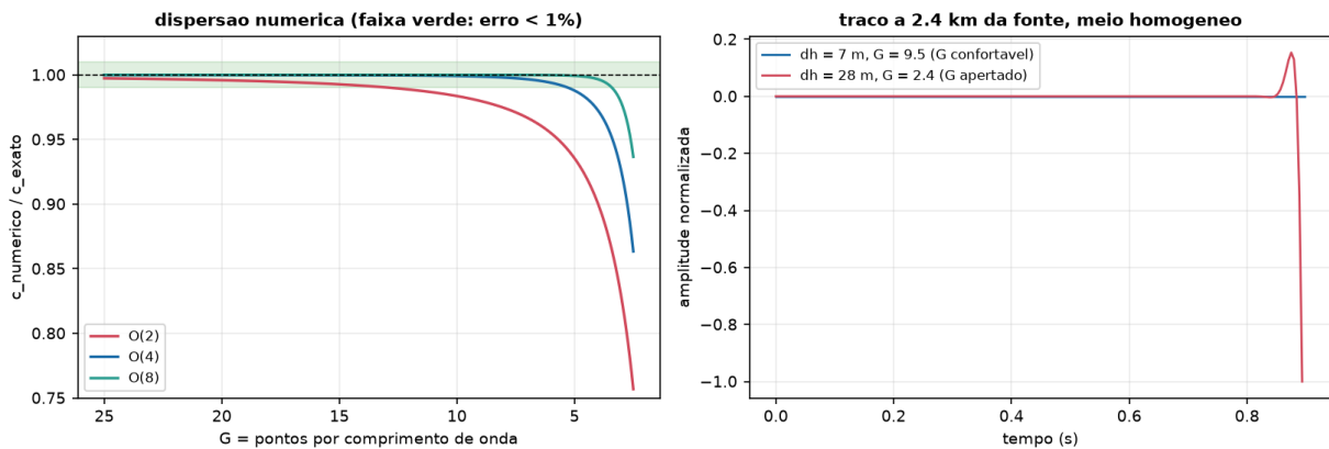
Figura 3.1: Esquerda: curva de dispersão numérica por ordem espacial. Direita: traço a 2,4 km da fonte em meio homogêneo, com G = 9,5 e G = 2,4 . A cauda no traço vermelho não existe na física.
