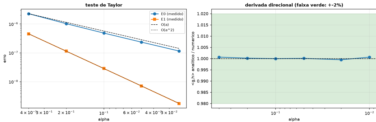
Figura 9.1: Esquerda: teste de Taylor em escala log-log, com as retas de referência \mathcal{O}(\alpha) e \mathcal{O}(\alpha^2) . Direita: razão da derivada direcional (faixa verde: \pm 2\% ).
