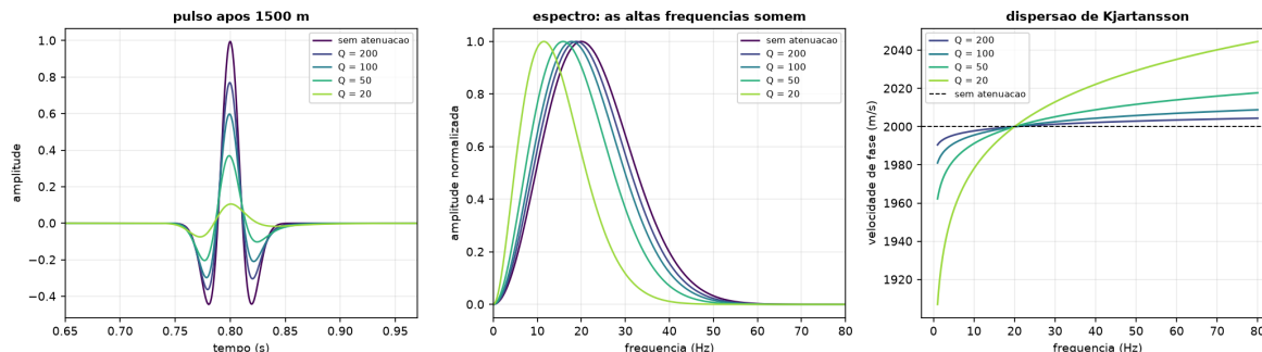
Figura 11.1: Modelo constant- Q : pulso, espectro e dispersão da velocidade de fase. Os três efeitos — perda de amplitude, descida da frequência de pico e mudança de velocidade — são inseparáveis, por causalidade.
