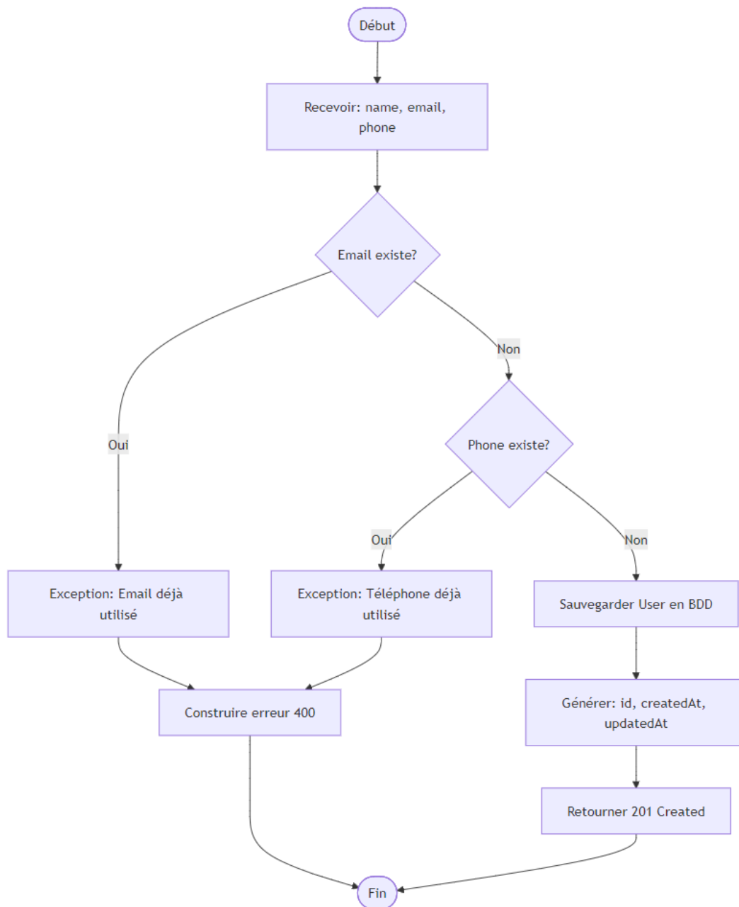
FIGURE 2 – Graphe de flux de contrôle - Création d'Utilisateur
