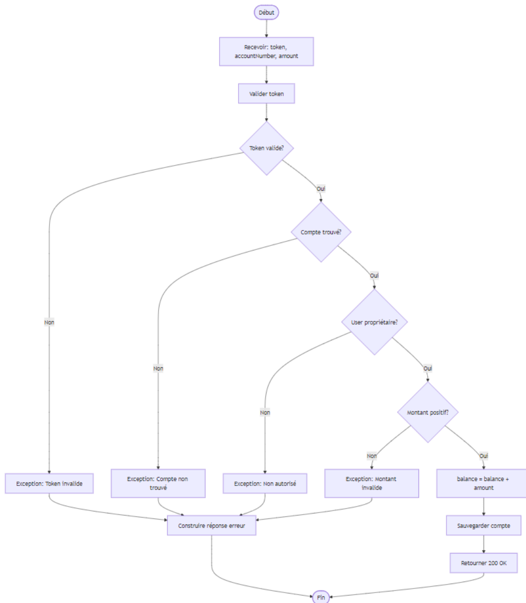
FIGURE 4 – Graphe de flux de contrôle - Dépôt
