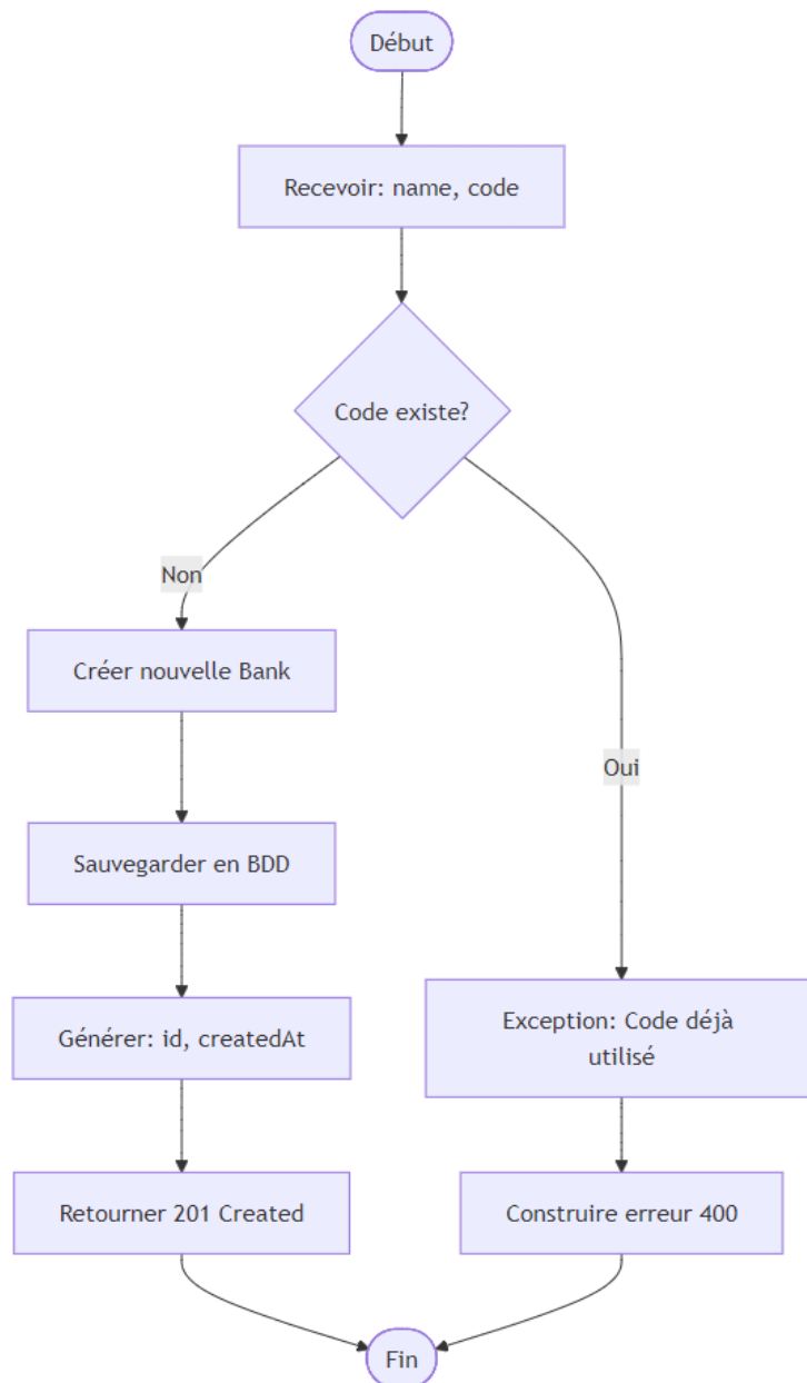
FIGURE 1 – Graphe de flux de contrôle - Création de Banque
