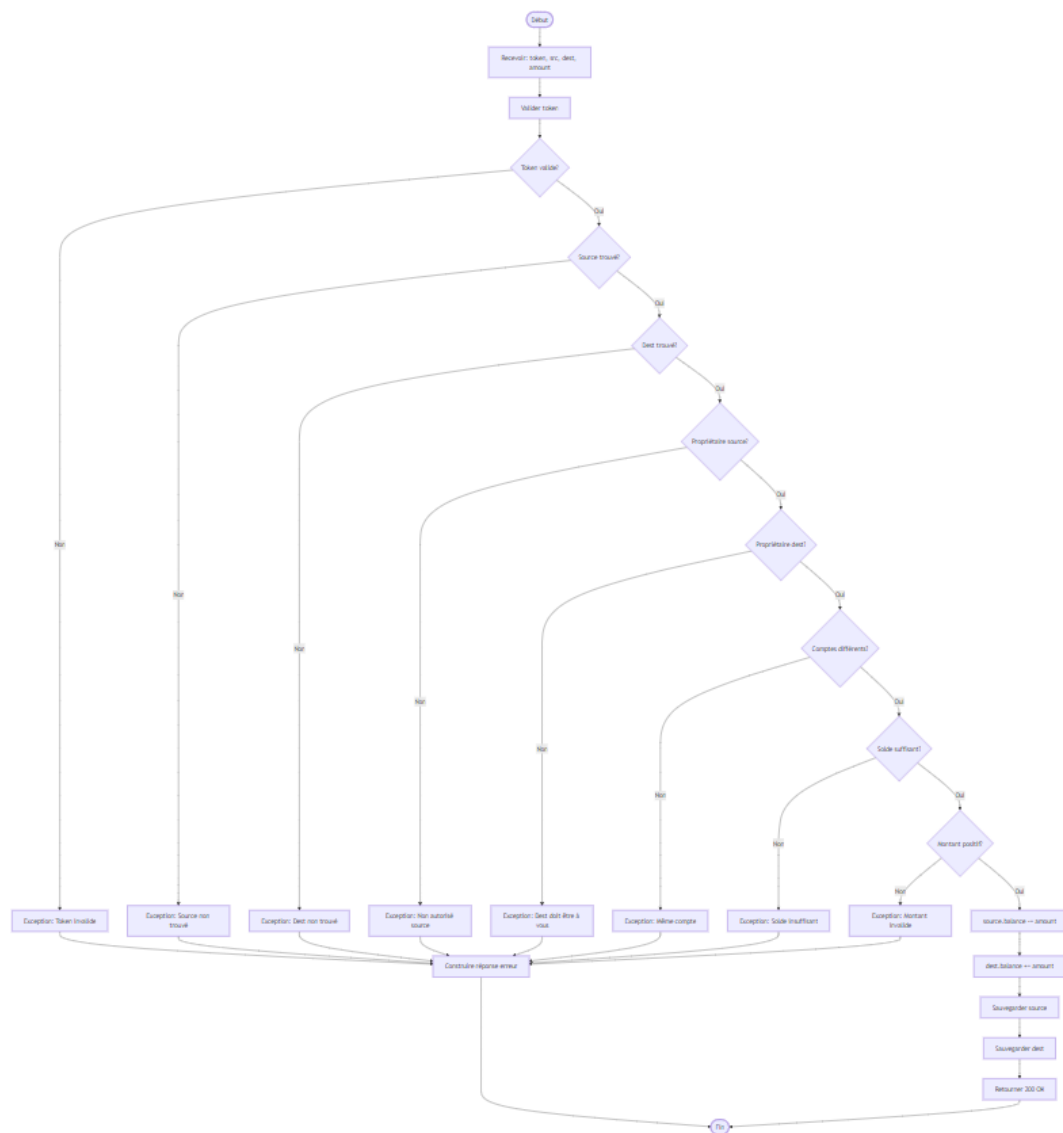
FIGURE 3 – Graphe de flux de contrôle - Transfert de Fonds
