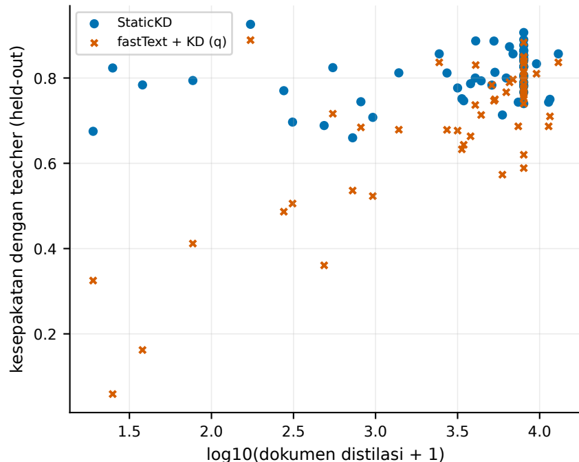
Held-out: kesepakatan per bahasa vs data
