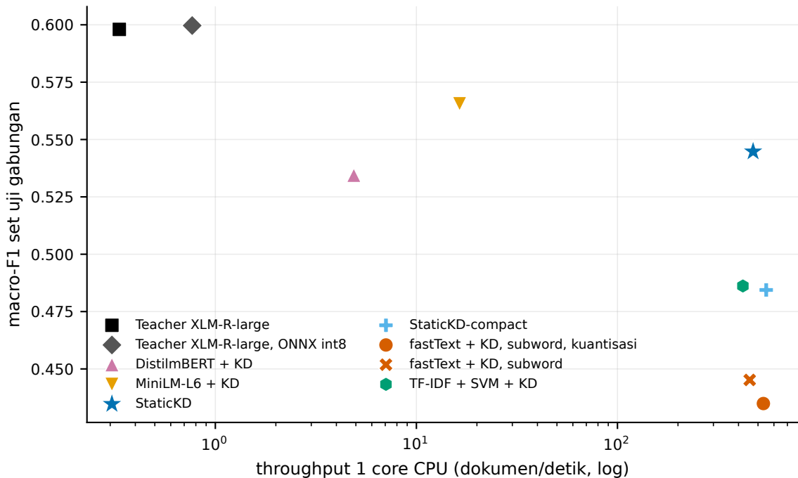
Trade-off akurasi-biaya
