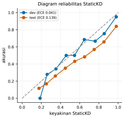
Gbr. 10. Diagram reliabilitas StaticKD pada dev dan set uji.
