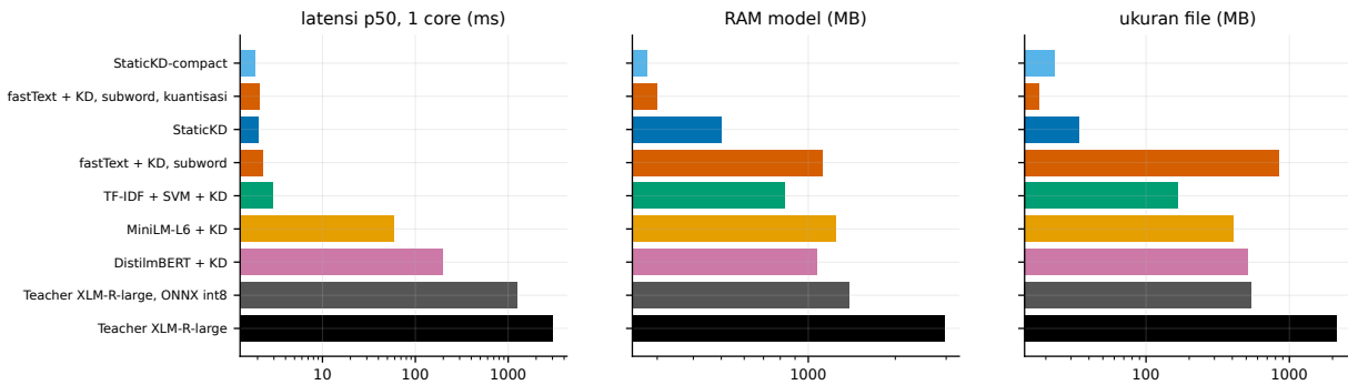
Gbr. 7. Latensi per artikel, RAM model, dan ukuran file (skala log).
