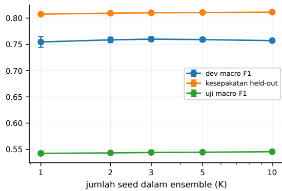
Gbr. 5. Pengaruh ukuran ensemble label (rata-rata \pm SD atas kombinasi seed ).
