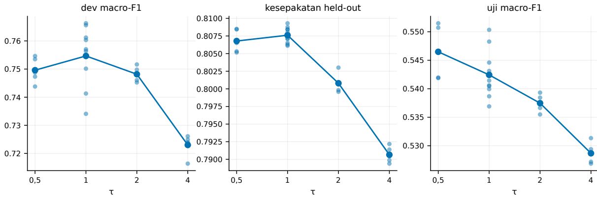
Gbr. 4. Pengaruh temperature distilasi. Titik = satu seed , garis = rata-rata.
