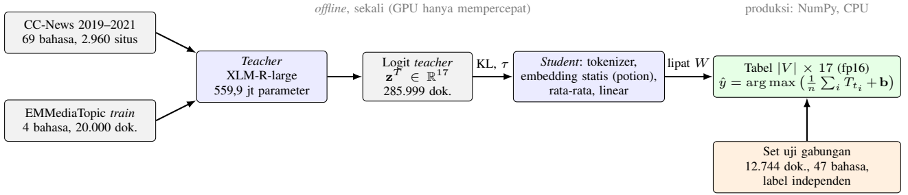
Gbr. 1. Alur StaticKD. Teacher melabeli korpus berita tak berlabel sekali secara offline ; student dilatih meniru distribusi teacher , lalu kepala linearnya dilipat ke dalam tabel token sehingga inferensi hanya berupa pengambilan baris tabel dan rata-rata. Evaluasi akhir memakai set uji yang labelnya independen dari teacher .
