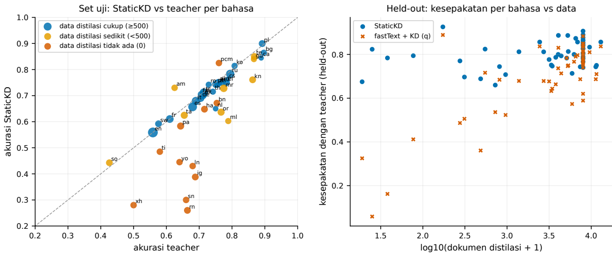
Gbr. 8. Kiri: akurasi StaticKD terhadap akurasi teacher per bahasa uji (warna = jumlah data distilasi bahasa, ukuran = jumlah artikel). Kanan: kesepakatan per bahasa held-out terhadap jumlah data distilasi, StaticKD vs fastText + KD.
