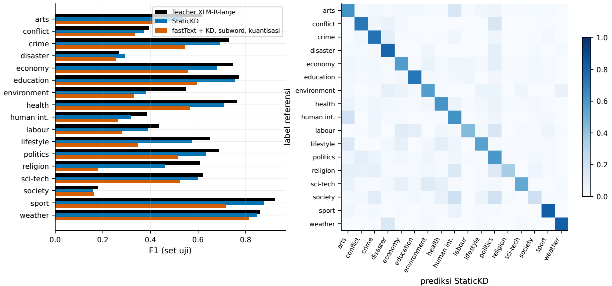
Gbr. 9. F1 per label di set uji (kiri) dan confusion matrix StaticKD yang dinormalisasi per label referensi (kanan).
