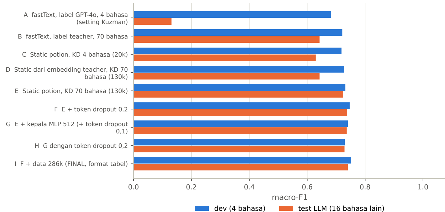
Ablasi komponen StaticKD
