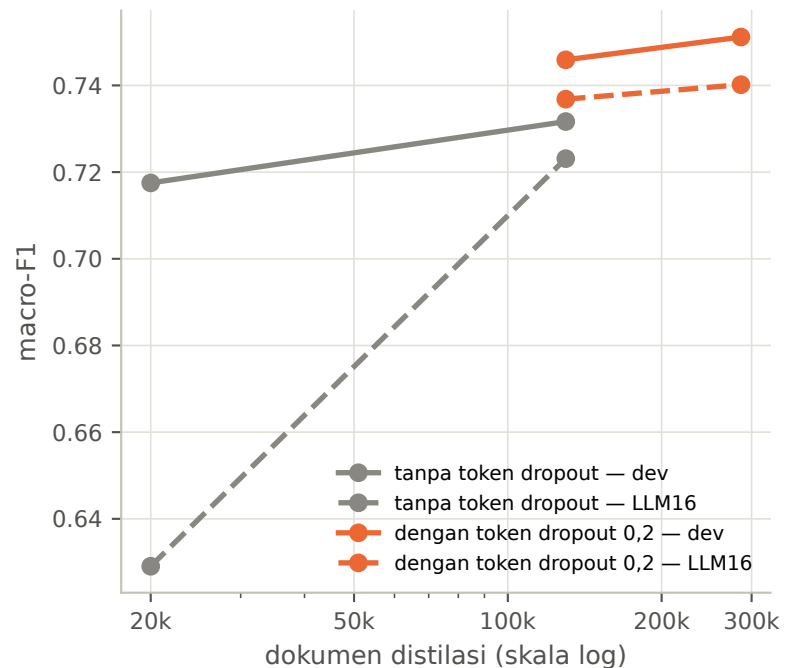
Skala data distilasi
