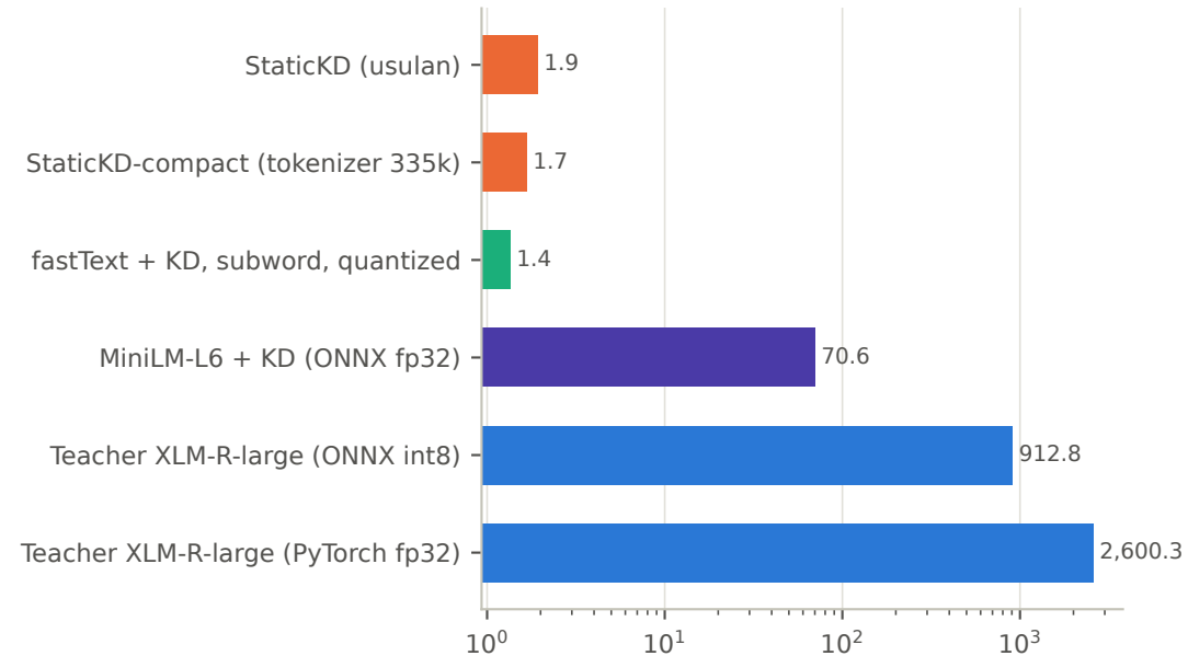
Latensi per artikel, 1 core (ms, log)
