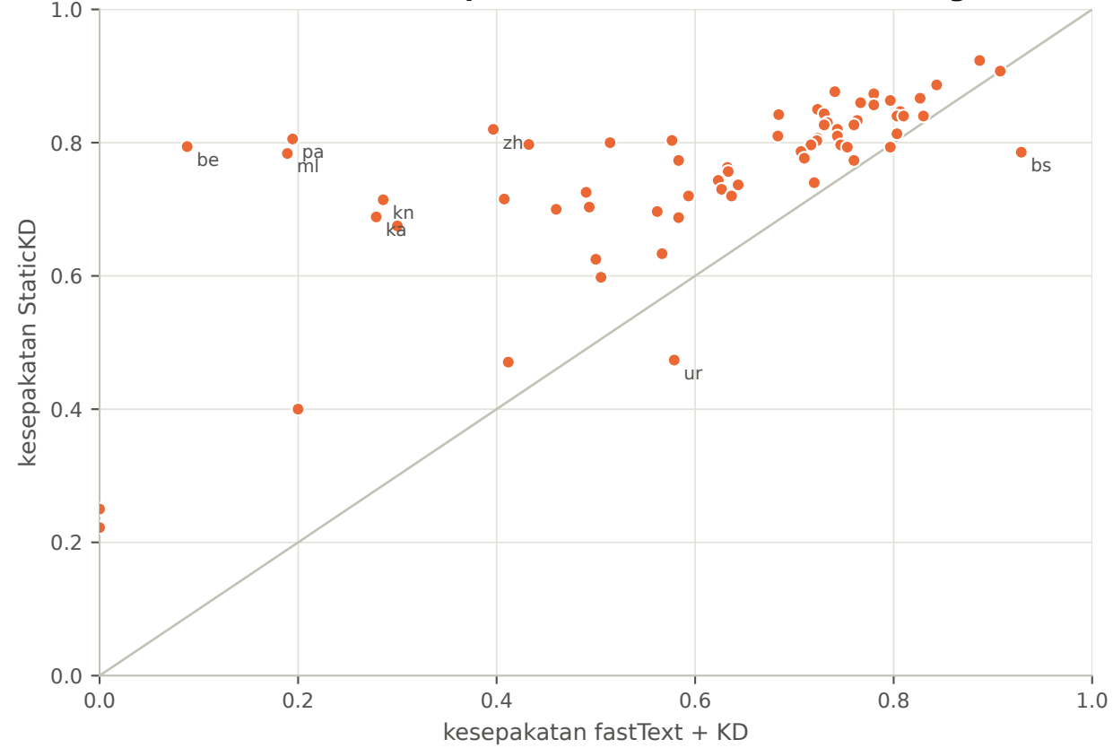
StaticKD vs fastText per bahasa (94% bahasa di atas garis)
