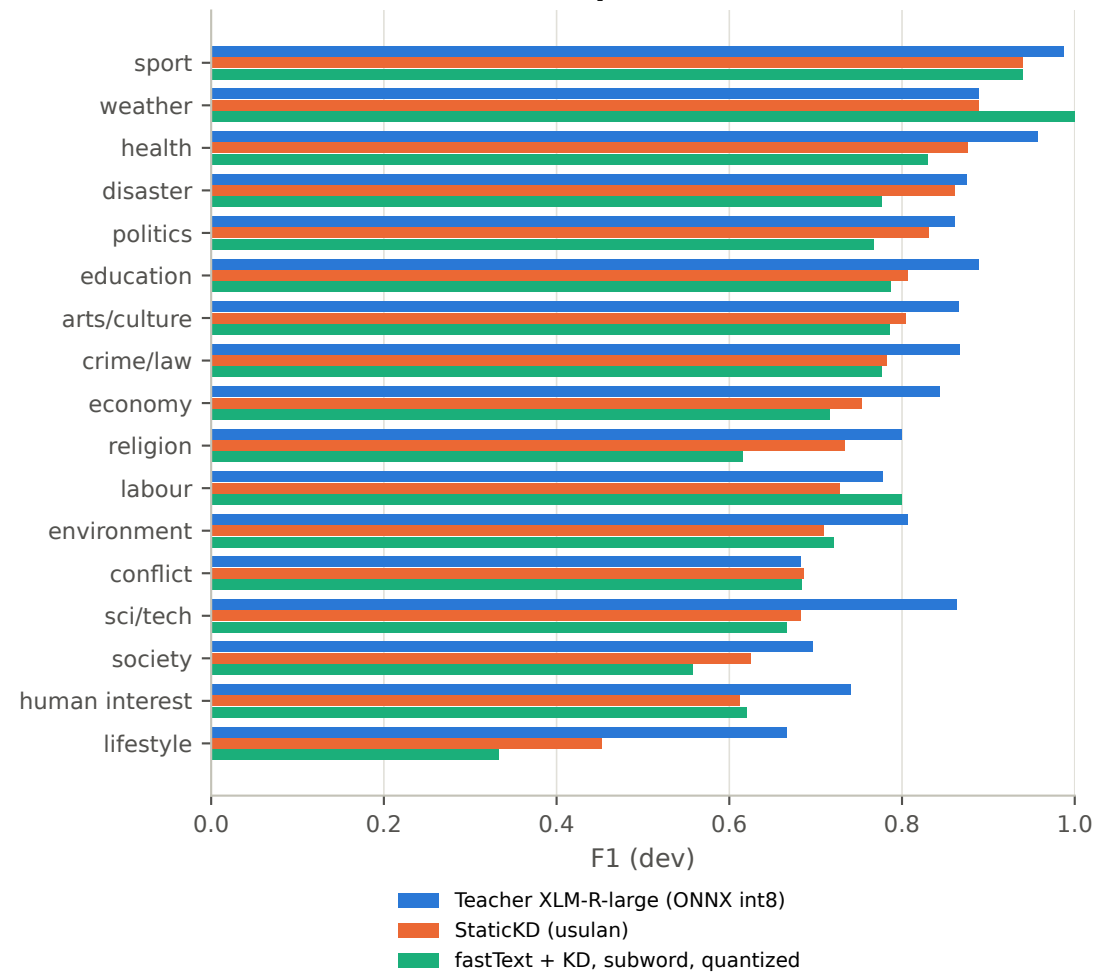
F1 per label
