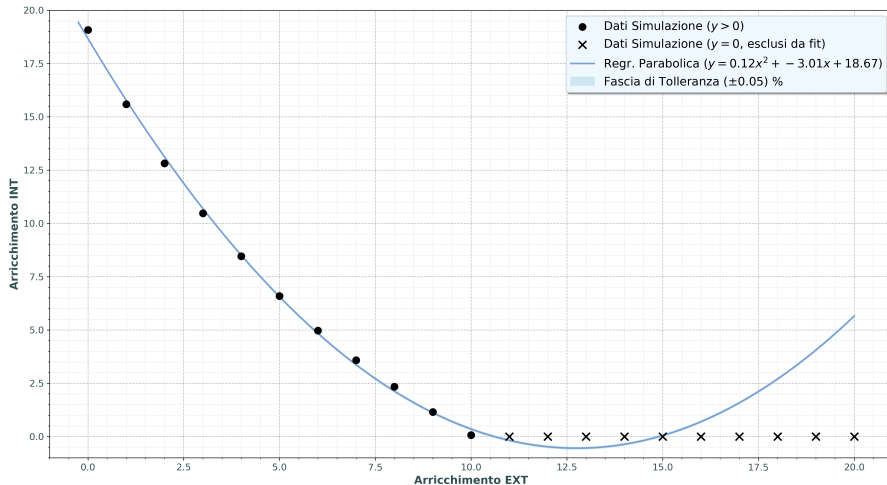
MAPPA DI STABILITÀ Regressione Parabolica: Arricchimento INT vs EXT Fit calcolato escludendo i punti con Arricchimento INT = 0 per matching k_{\max} = 0.97547 con pitch = x1
