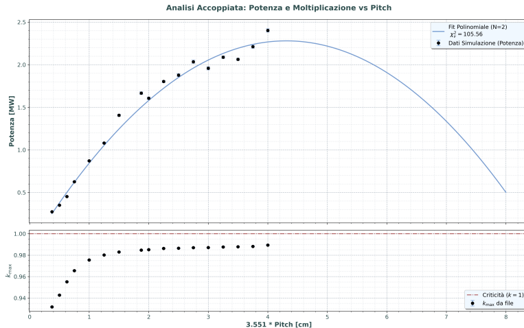
Figure: Caratterizzazione delle prestazioni del core: correlazione tra il fattore di moltiplicazione k_{\max} e
