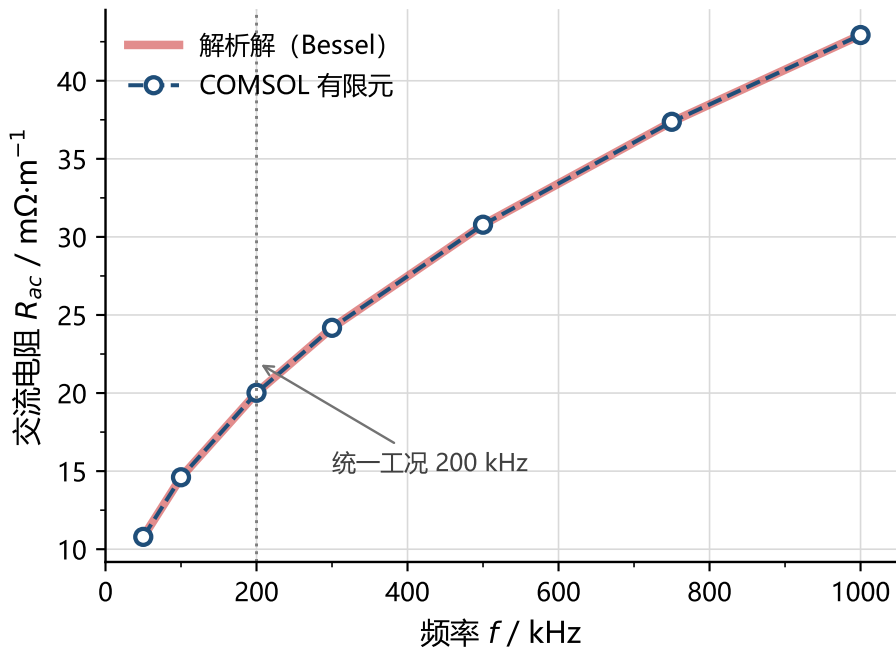
(a) 交流电阻的频率特性
