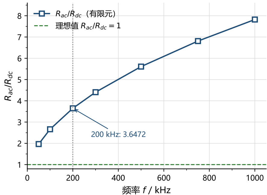
(b) 交直流电阻比的频率特性
