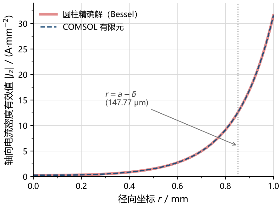
(a) 电流密度的径向分布
