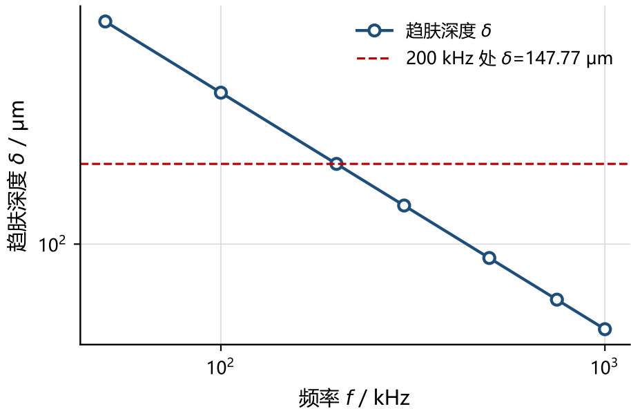
铜的趋肤深度随频率的变化
