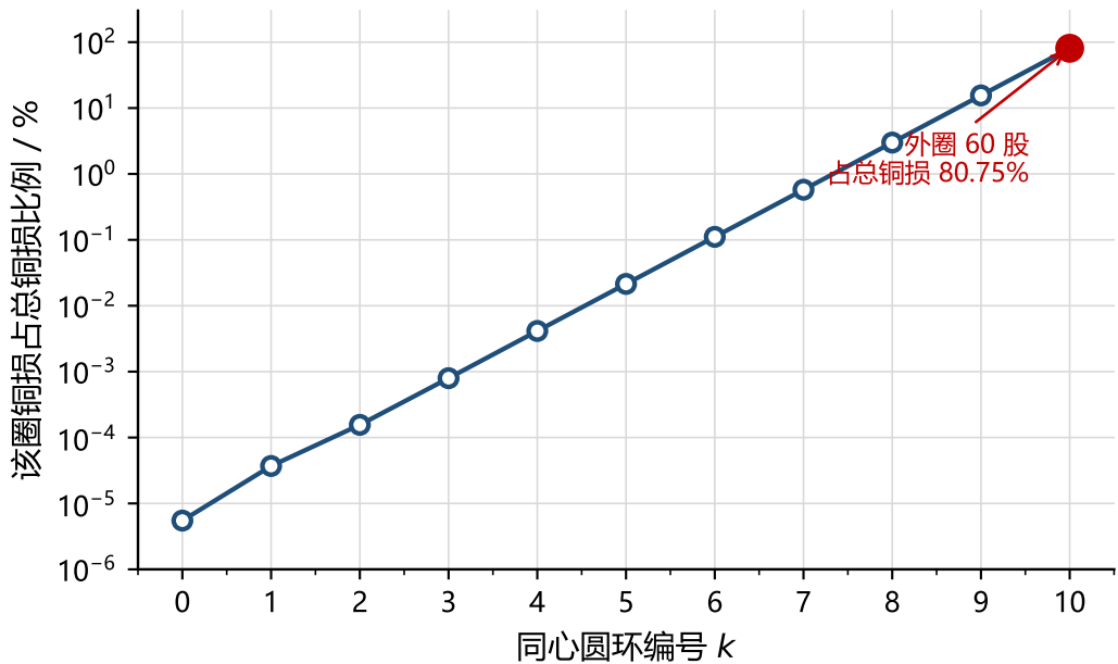
铜损沿径向的高度集中
