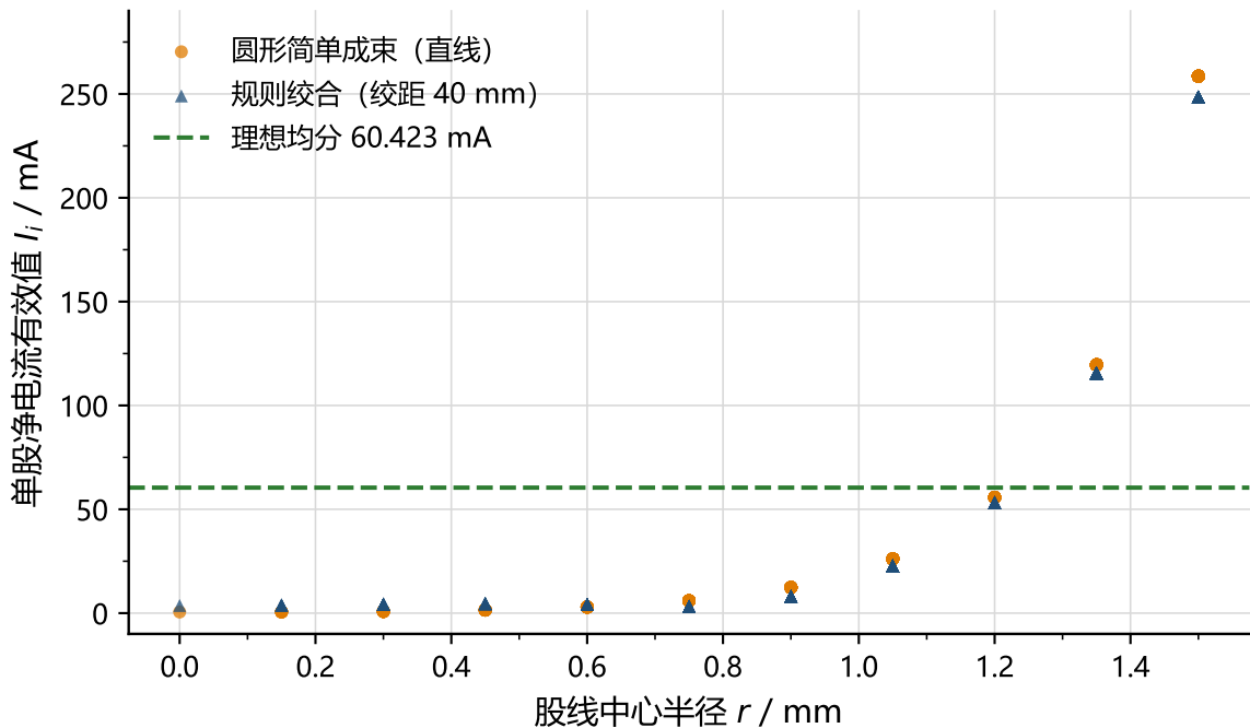
两种结构下股电流沿径向的分布对照
