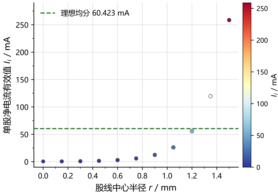
(a) 331 股电流沿径向的分布
