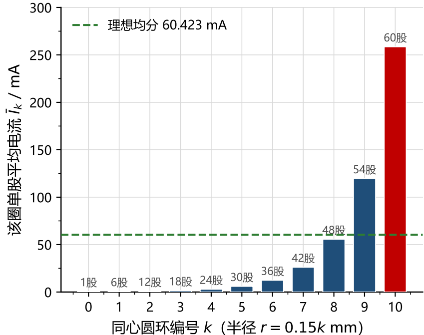
(b) 各同心圆环的平均股电流
