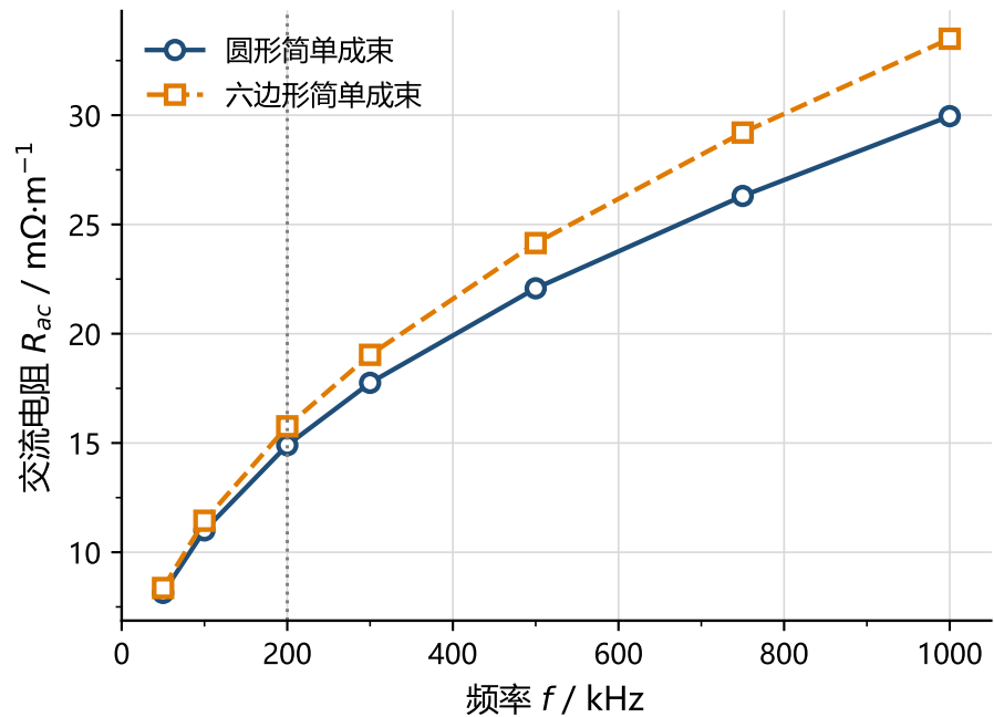
(b) 两种排布方式的频率响应
