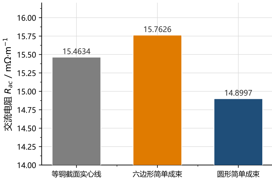
(a) 三种结构的交流电阻
