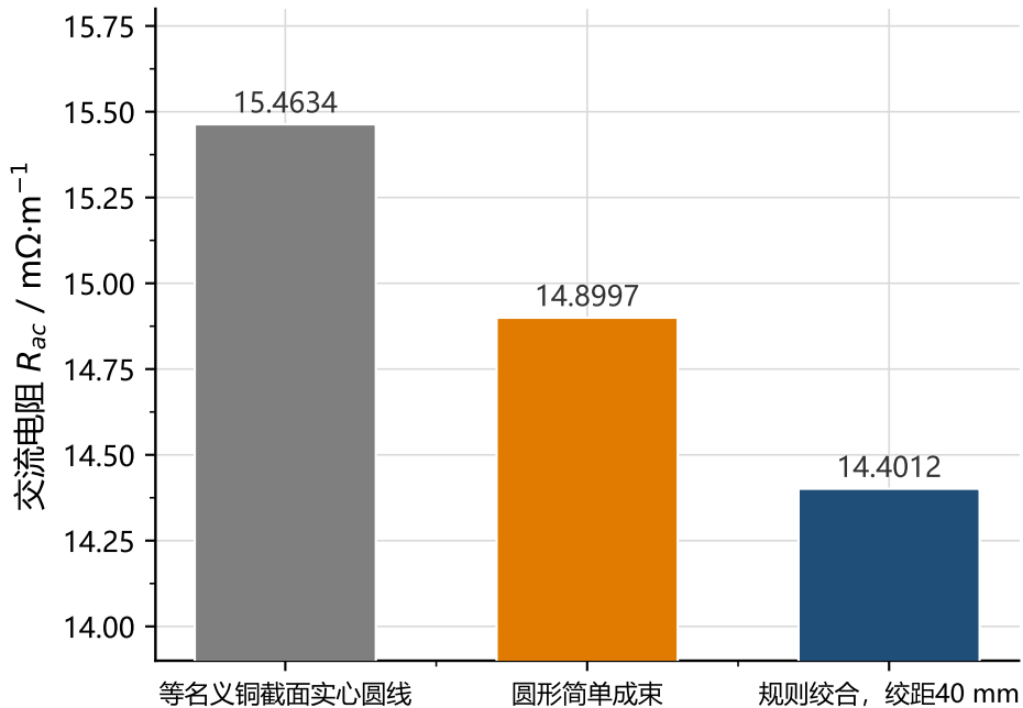
(a) 三方案交流电阻对照
