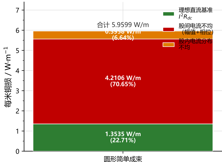
(b) 圆形成束铜损的构成分解
