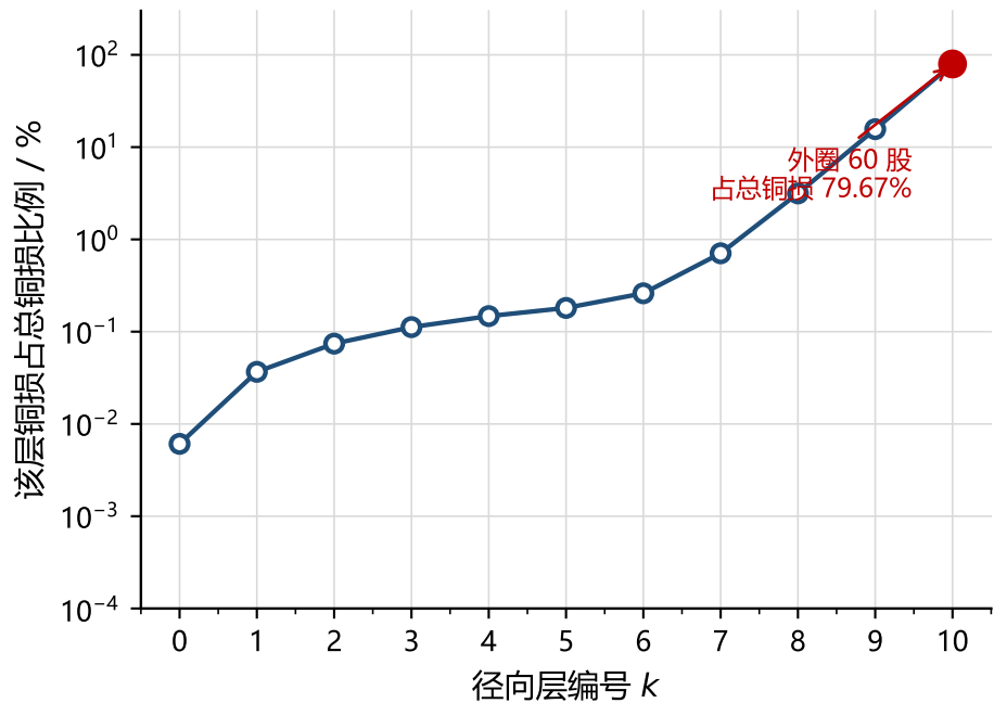
(b) 规则绞合：铜损的径向集中
