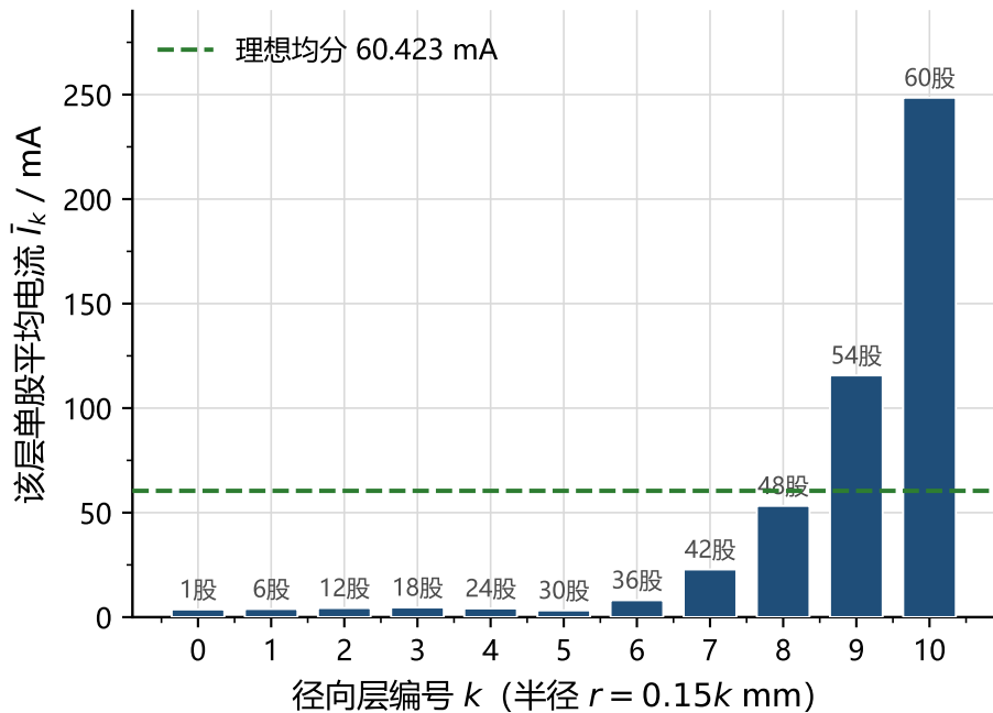
(a) 规则绞合：分层平均电流
