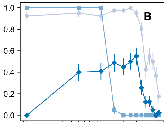
Lotka-Volterra
