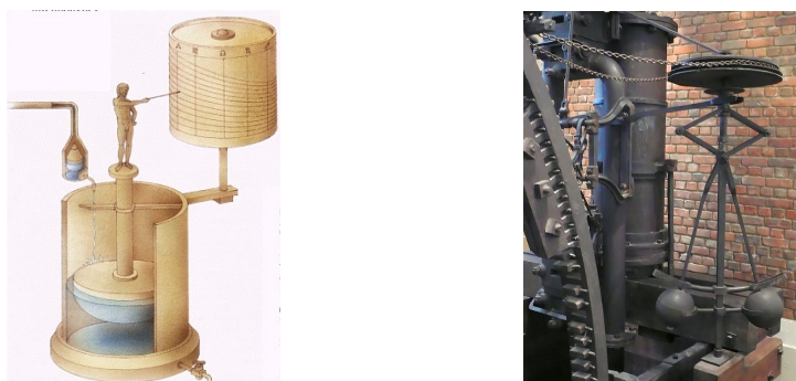
FIGURE 1.1 – À gauche, la clepsydre de Ctésibios et son régulateur à flotteur. À droite, le régulateur à boules de Watt sur une machine de Boulton & Watt.
