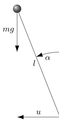
FIGURE 1.3 – Pendule inversé contrôlé.
