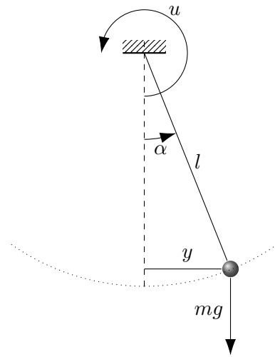
FIGURE 1.2 – Pendule simple contrôlé.
