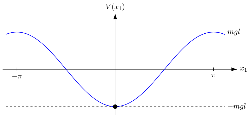
FIGURE 2.7 – Énergie potentielle du pendule, V(x_1) = -mgl \cos x_1 . La position basse x_1 = 0 est un minimum (puits de potentiel), les positions hautes x_1 = \pm\pi des maxima. Une fonction de Lyapunov pour (0, 0) s'obtient en ajoutant à V l'énergie cinétique.
