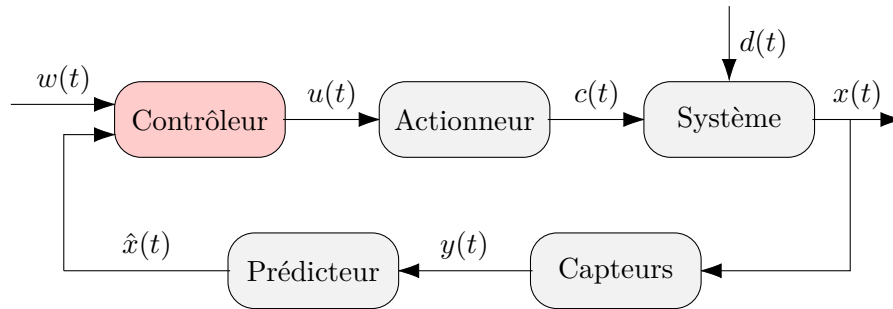
FIGURE 1.7 – Schéma fonctionnel complet d'un système en boucle fermée.
