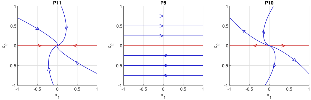
FIGURE 2.3 – A non diagonalisable, valeur propre double \lambda . À gauche \lambda < 0 (nœud impropre puits), au milieu \lambda = 0 , à droite \lambda > 0 (nœud impropre source) : cas P_{11} , P_5 et P_{10} du TD1.
