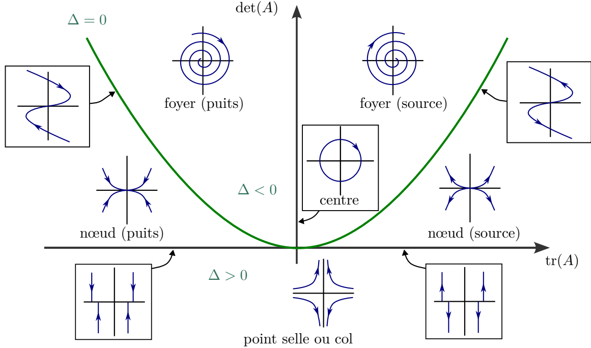
FIGURE 2.4 – Diagramme de bifurcation dans le plan (\text{tr}(A), \det(A)) pour \dot{x}(t) = Ax(t) , n = 2 . La parabole \Delta = \text{tr}(A)^2 - 4\det(A) = 0 sépare les valeurs propres réelles ( \Delta \geq 0 ) des valeurs propres complexes ( \Delta < 0 ) ; la moitié gauche ( \text{tr}(A) < 0 ) correspond aux équilibres asymptotiquement stables. Le TD1 y place les onze cas P_1 à P_{11} , dont les portraits de phase sont ceux des Figures 2.1 à 2.3.
