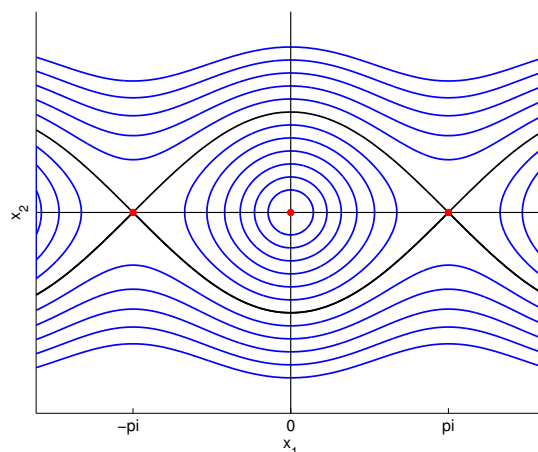
FIGURE 2.6 – Portrait de phase du pendule simple non amorti. L'équilibre (0,0) (position basse) est stable mais non asymptotiquement stable : les orbites voisines sont des courbes fermées. Les équilibres (\pm\pi,0) (position haute) sont instables et reliés par des trajectoires hétéroclines . Avec frottement, (0,0) devient asymptotiquement stable.
