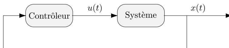
FIGURE 1.5 – Schéma fonctionnel simple d'un système en boucle fermée.
