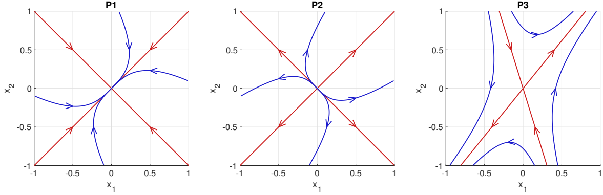
FIGURE 2.1 – A diagonalisable dans \mathbb{R} . À gauche \lambda_1, \lambda_2 < 0 (nœud puits), au milieu \lambda_1, \lambda_2 > 0 (nœud source), à droite \lambda_1 \lambda_2 < 0 (col) : cas P_1, P_2 et P_3 du TD1.
