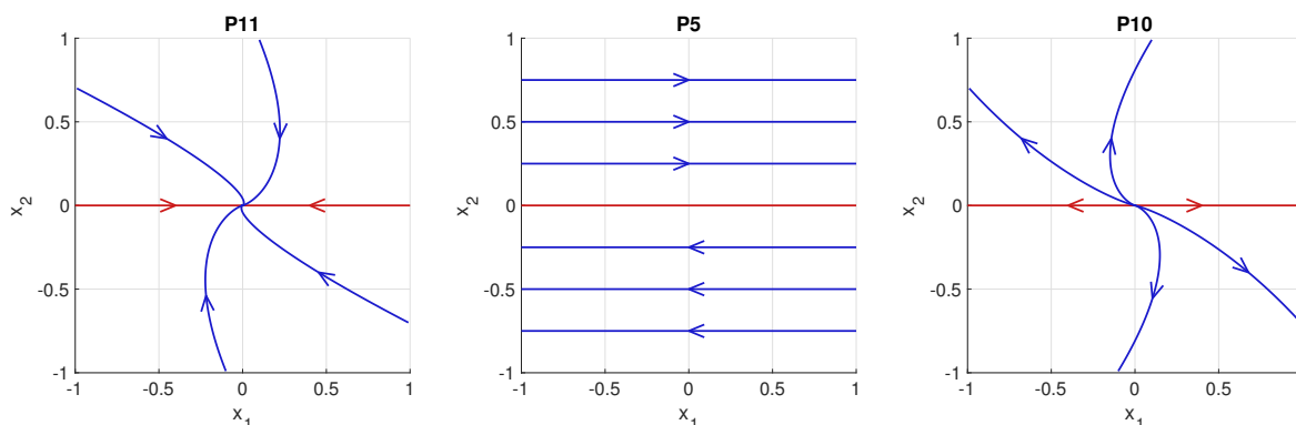
FIGURE 2.3 – A non diagonalisable, valeur propre double \lambda . À gauche \lambda < 0 (nœud impropre puits), au milieu \lambda = 0 , à droite \lambda > 0 (nœud impropre source) : cas P_{11} , P_5 et P_{10} du TD1.
