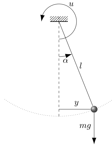
FIGURE 1.2 – Pendule simple contrôlé.
