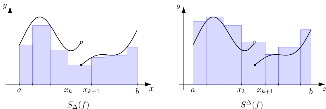
FIGURE 1.1 – Sommes de Darboux inférieure (à gauche) et supérieure (à droite) d'une fonction discontinue, associées à une subdivision non régulière.
