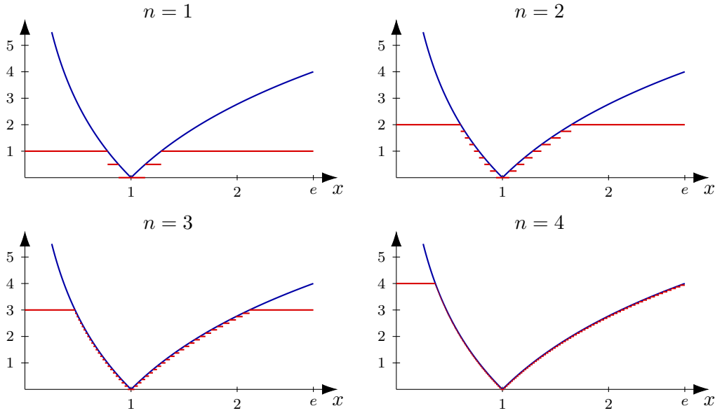
FIGURE 3.1 – Approximation de f(x) = 4|\ln x| sur [0, e] , avec f(0) = +\infty , par la suite croissante (f_n) de fonctions étagées construite dans la preuve du Théorème 3.2.1. De gauche à droite et de haut en bas, on a n = 1, 2, 3 et 4 .
