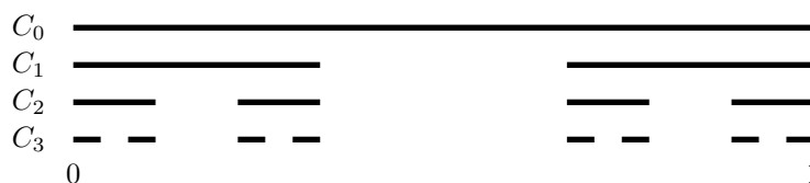
FIGURE 2.2 – Les quatre premières étapes C_0, C_1, C_2, C_3 de la construction de l'ensemble de Cantor : à chaque étape, on retire le tiers central ouvert de chaque segment.
