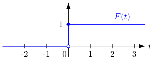
FIGURE 2.1 – Représentation graphique de la fonction de répartition pour la mesure de Dirac en 0, \delta_0 , qui dans ce cas est la fonction de Heaviside.
