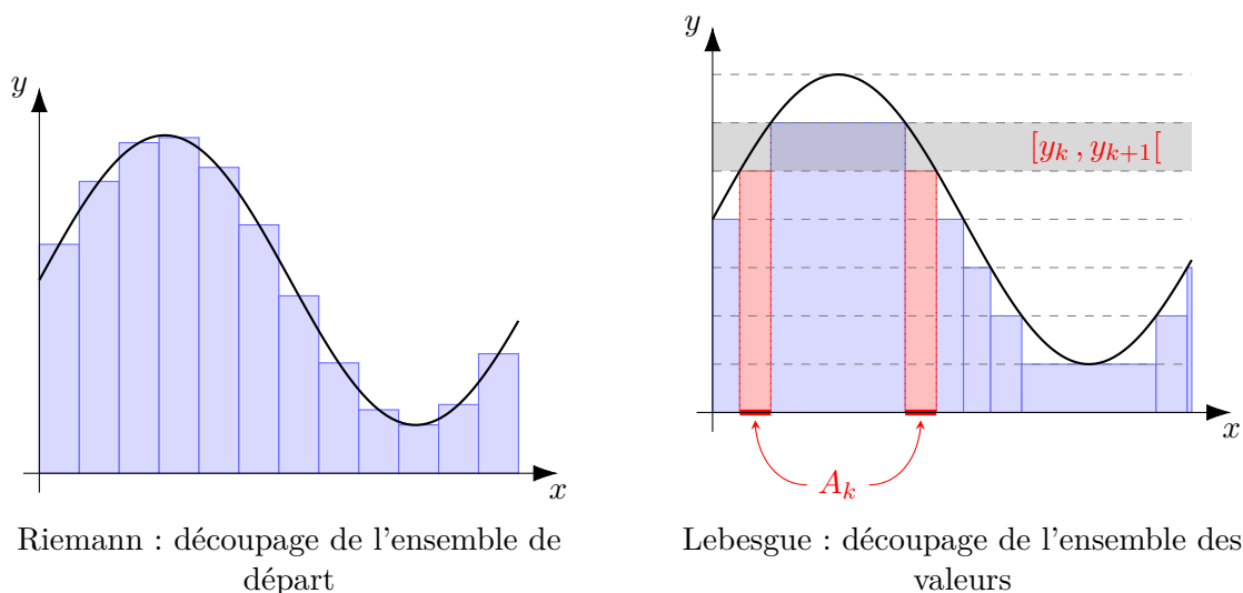
FIGURE 1.2 – Les deux découpages. À gauche, f est approchée par une constante sur chaque petit intervalle ; à droite, par la valeur y_k sur chaque ensemble de niveau. L'ensemble A_k des points où f prend ses valeurs dans la bande [y_k, y_{k+1}[ est ici réunion de deux intervalles : il contribue à l'intégrale par les deux rectangles rouges, de hauteur y_k .
