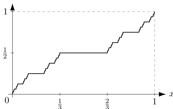
FIGURE B.1 – L'escalier de Cantor : une fonction continue et croissante de 0 à 1, constante sur chacun des intervalles retirés pour construire l'ensemble de Cantor.
