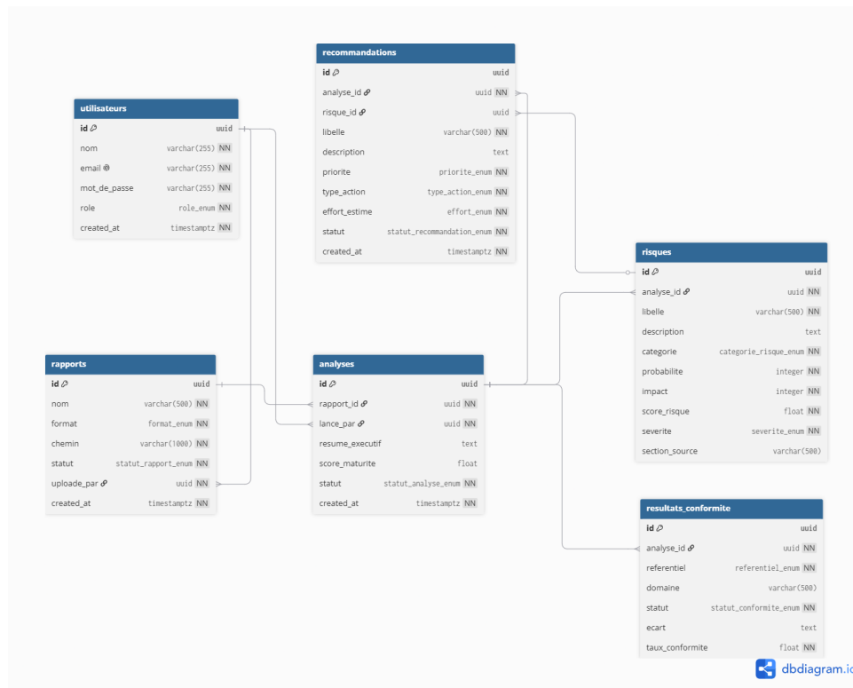
FIGURE 4.3 – Schéma physique PostgreSQL — tables et clés étrangères
