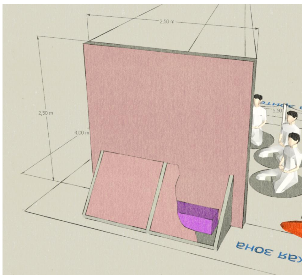
Рисунок 11. Эскиз конструкции скульптуры (фиолетовый блок – утяжелитель)
