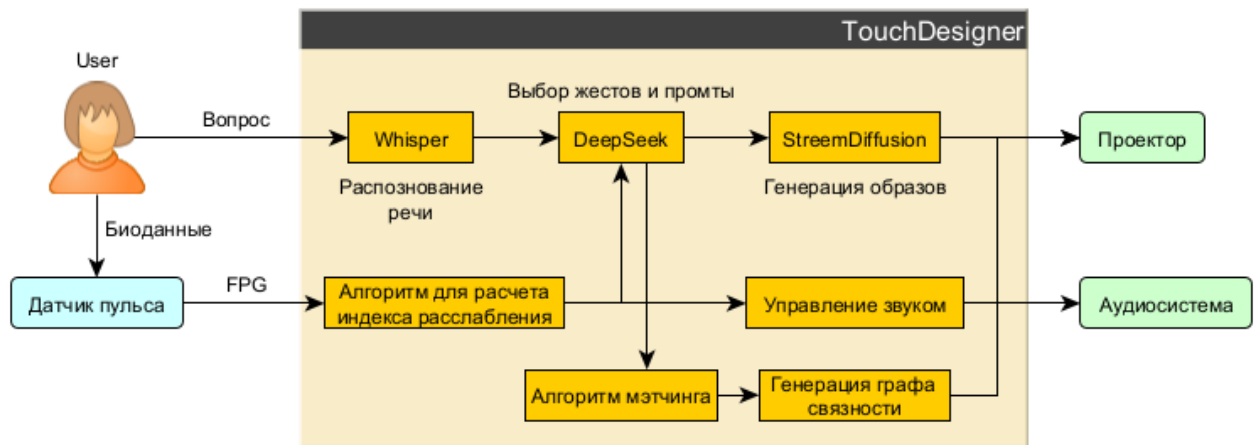
Рисунок 9. Схема генерации контента
