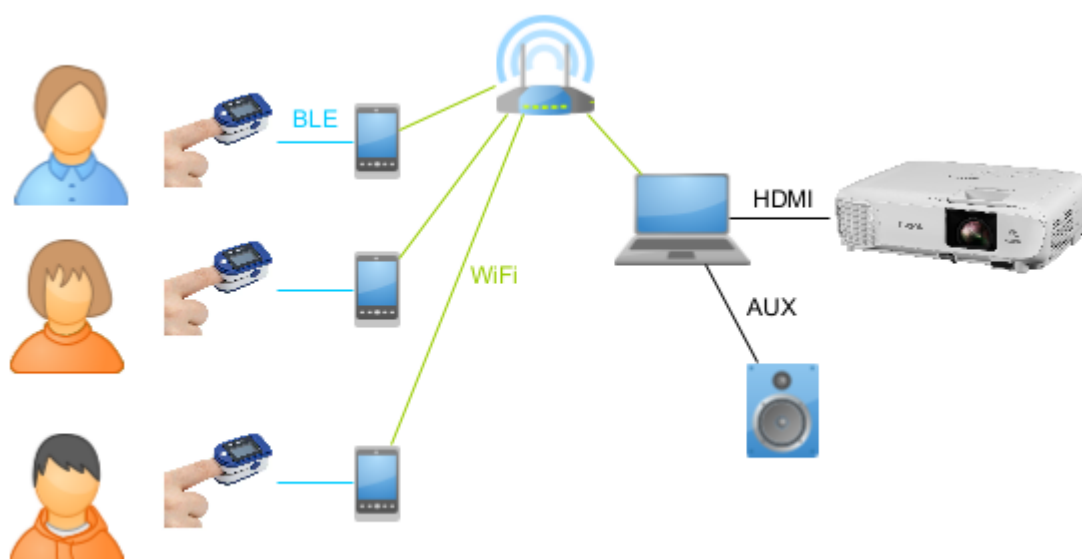
Рисунок 6. Схема подключения
