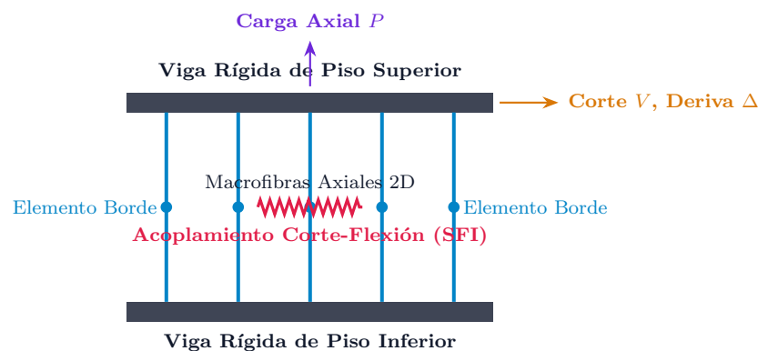
Figura 3: Formulación del macroelemento bidimensional de interacción corte-flexión SFI-MVLEM.
