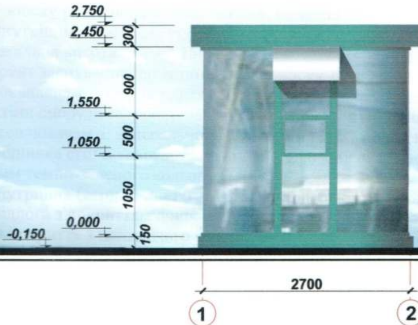
Бічний фасад
